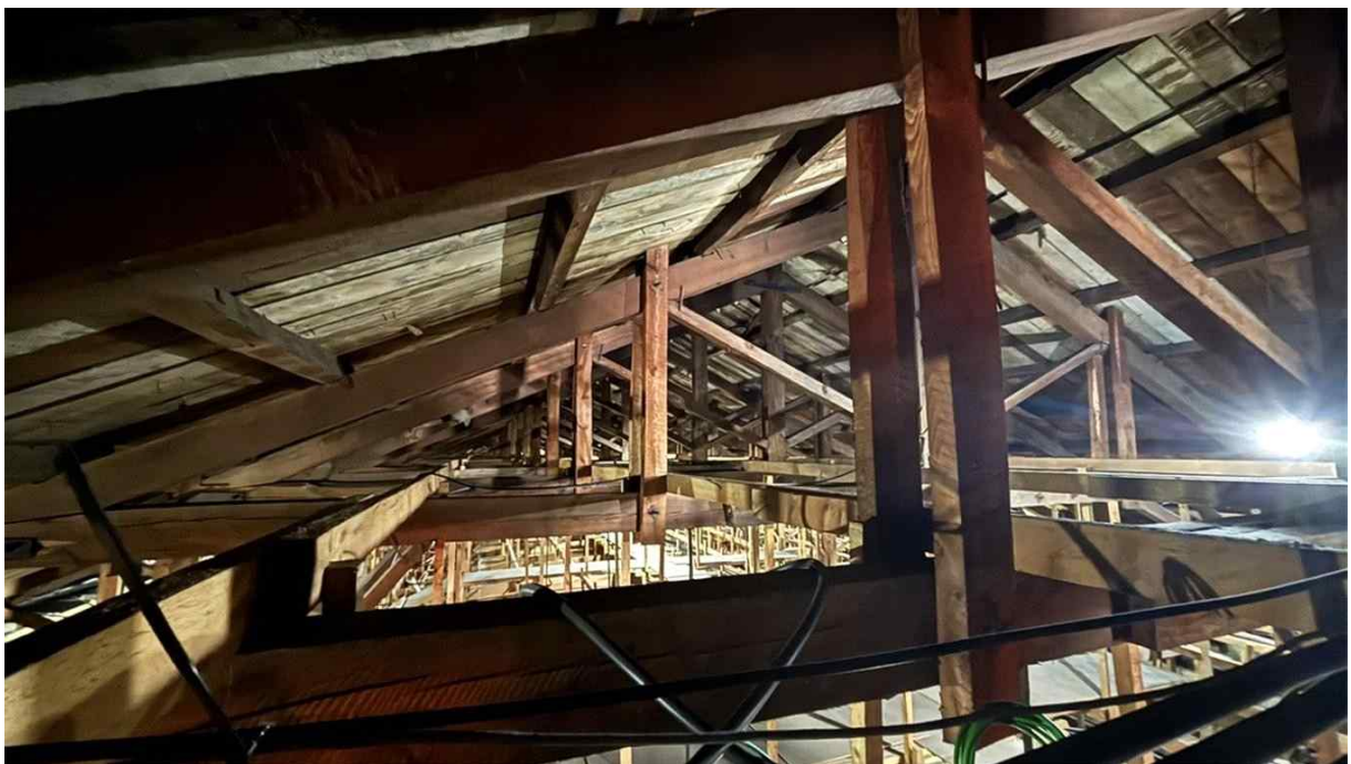
< 「전주 중앙성당」의 필수보존요소 ‘지붕 트러스 구조’ >
